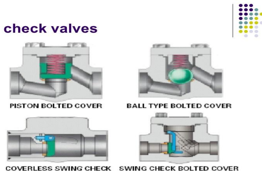
Fig: Check Valves
